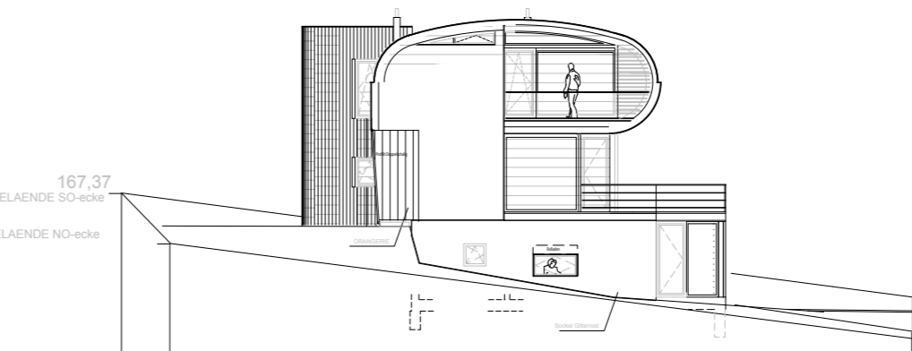
ANSICHT SÜDEN
