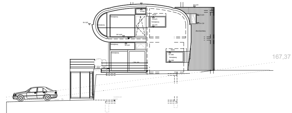
ANSICHT SÜDEN
