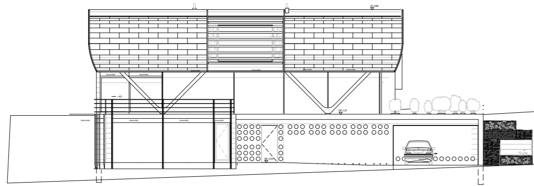
ANSICHT WESTEN
