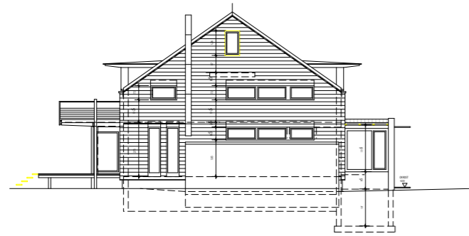
ANSICHT OST
