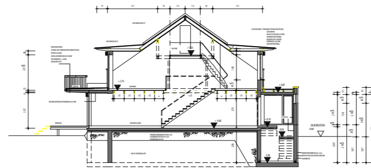
SCHNITT 1-1
