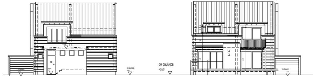
ANSICHT NORD
