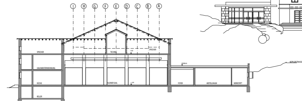
SCHNITT B - B
