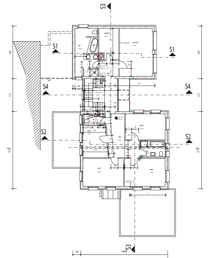
OBERGESCHOSS
